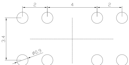
P.C.B LAND DIMENSION
