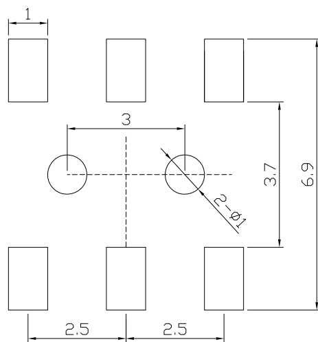
P.C.B LAND DIMENSION
