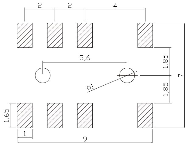
P.C.B. LAYOUT
