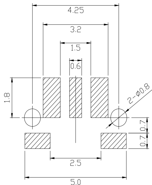
P.C.B LAND DIMENSION
